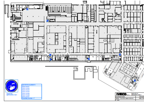
Lay-out Posizionamento dei dispenser
